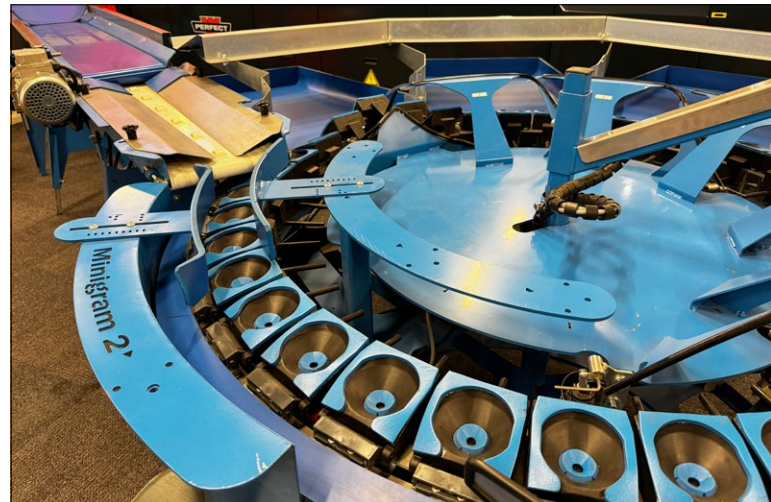
De ronde CALIBREX Minigram sorteermachine is leverbaar in een versie met grote cups voor de sortering van pitfruit of kleine cups voor steenfruit.
